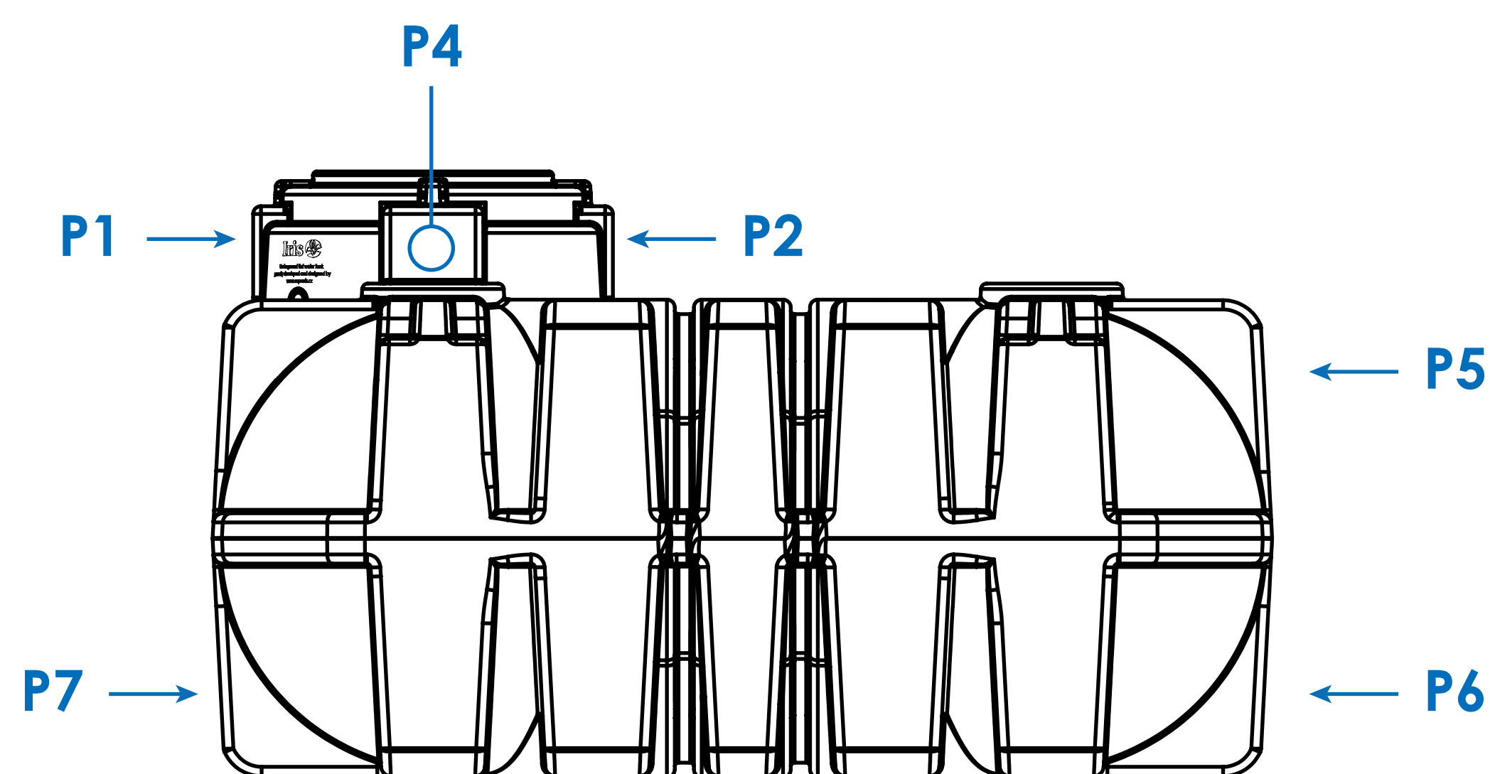
Boční pohled
